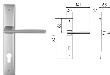
1030 MANIGLIA PER PORTA CON PIASTRA door-handle on back plate
