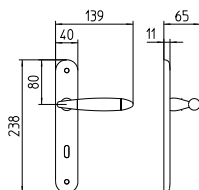
460 MANIGLIA PER PORTA CON PIASTRA door-handle on back plate
