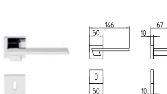
1371 MANIGLIA PER PORTA CON ROSETTA door-handle on rose
