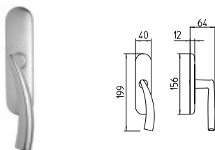
772/M CREMONESE IMPUGNATURA MANIGLIA window lever-handle
