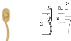
712/DK MARTELLINA DK drehkipp system
