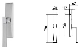
1172/M CREMONESE IMPUGNATURA MANIGLIA window lever-handle
