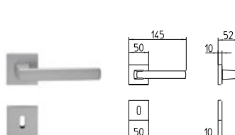
1291 MANIGLIA PER PORTA CON ROSETTA door-handle on rose
