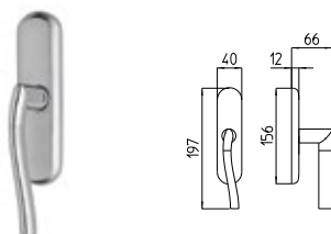
1182/M CREMONESE IMPUGNATURA MANIGLIA window lever-handle
