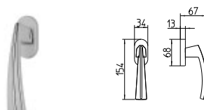
1142/DK MARTELLINA DK drehkipp system
