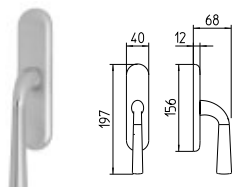
S102/M CREMONESE IMPUGNATURA MANIGLIA window lever-handle
