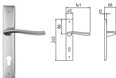
1480 MANIGLIA PER PORTA CON PIASTRA door-handle on back plate
