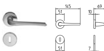
1491 MANIGLIA PER PORTA CON ROSETTA door-handle on rose
