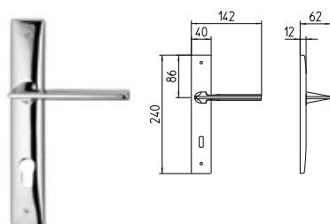
1460 MANIGLIA PER PORTA CON PIASTRA door-handle on back plate
