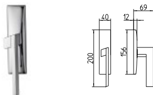
1372/M CREMONESE IMPUGNATURA MANIGLIA window lever-handle
