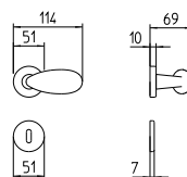
1091 MANIGLIA PER PORTA CON ROSETTA door-handle on rose
