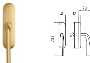
722/M CREMONESE IMPUGNATURA MANIGLIA window lever-handle
