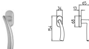
772/DK MARTELLINA DK drehkip system
