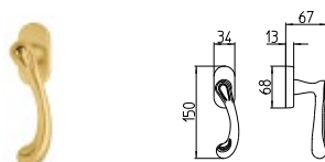
542/DK MARTELLINA DK drehkipp system
