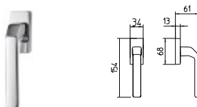
1602/DK MARTELLINA DK drehkipp system
