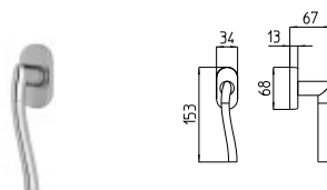
1182/DK MARTELLINA DK drehkipp system
