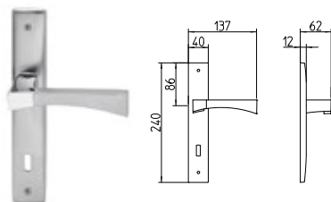
1170 MANIGLIA PER PORTA CON PIASTRA door-handle on back plate
