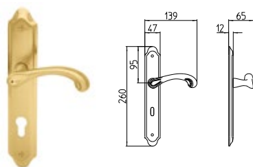
540 MANIGLIA PER PORTA CON PIASTRA door-handle on back plate
