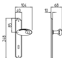
1110 MANIGLIA PER PORTA CON PIASTRA door-handle on back plate
