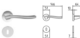
1481 MANIGLIA PER PORTA CON ROSETTA door-handle on rose
