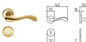
451 MANIGLIA PER PORTA CON ROSETTA door-handle on rose
