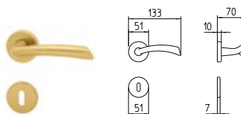
S61 MANIGLIA PER PORTA CON ROSETTA door-handle on rose
