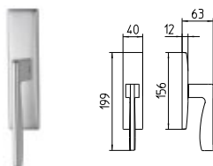
1032/M CREMONESE IMPUGNATURA MANIGLIA window lever-handle
