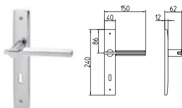
3180 MANIGLIA PER PORTA CON PIASTRA door-handle on back plate
