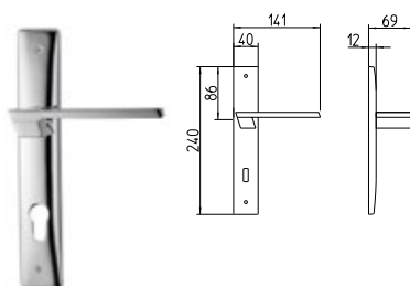
1370 MANIGLIA PER PORTA CON PIASTRA door-handle on back plate
