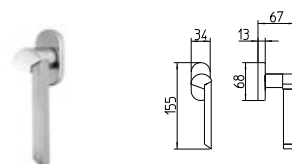
1152/DK MARTELLINA DK drehkipp system
