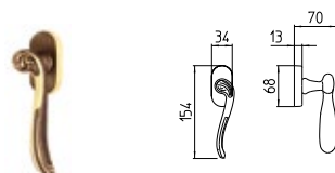
1022/DK MARTELLINA DK drehkipp system
