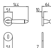
461 MANIGLIA PER PORTA CON ROSETTA door-handle on rose
