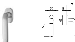
1612/DK MARTELLINA DK drehkipp system
