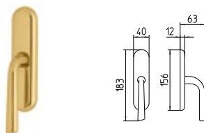
S62/M CREMONESE IMPUGNATURA MANIGLIA window lever-handle
