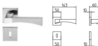
1171 MANIGLIA PER PORTA CON ROSETTA door-handle on rose
