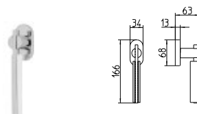
3182/DK MARTELLINA DK drehkipp system
