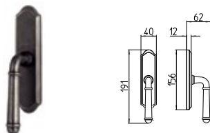
1342/M CREMONESE IMPUGNATURA MANIGLIA window lever-handle
