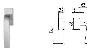
1502/DK MARTELLINA DK drehkipp system
