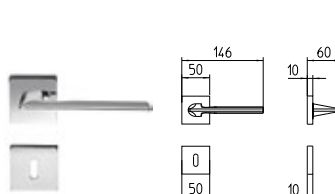
1461 MANIGLIA PER PORTA CON ROSETTA door-handle on rose
