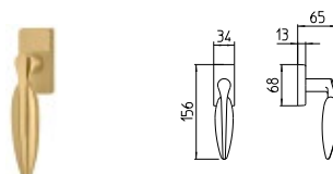
3122/DK MARTELLINA DK drehkipp system
