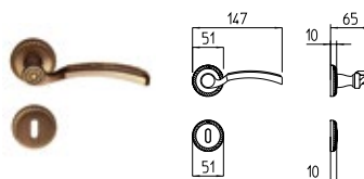
1411 MANIGLIA PER PORTA CON ROSETTA door-handle on rose
