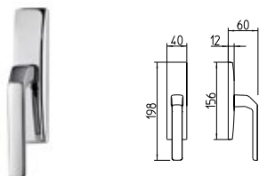
1602/M CREMONESE IMPUGNATURA MANIGLIA window lever-handle
