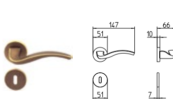
1221 MANIGLIA PER PORTA CON ROSETTA door-handle on rose
