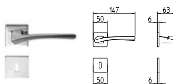
1631 MANIGLIA PER PORTA CON ROSETTA door-handle on rose
