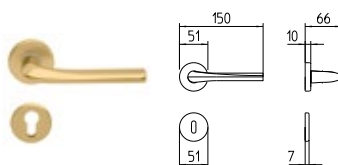
721 MANIGLIA PER PORTA CON ROSETTA door-handle on rose
