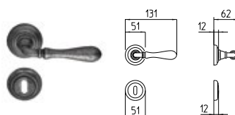
1421 MANIGLIA PER PORTA CON ROSETTA door-handle on rose
