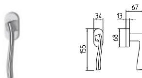
1482/DK MARTELLINA DK drehkipp system
