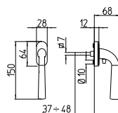
S102/DKM-SIC MARTELLINA DK MAGNETICO DI SICUREZZA security DK lever system
