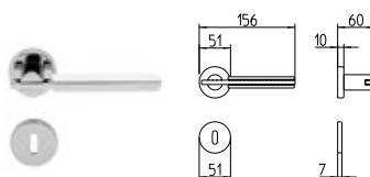
3181 MANIGLIA PER PORTA CON ROSETTA door-handle on rose
