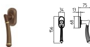
1512/DK MARTELLINA DK drehkipp system
