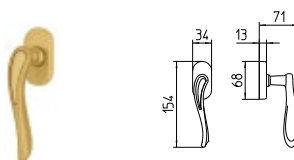
1012/DK MARTELLINA DK drehkipp system
