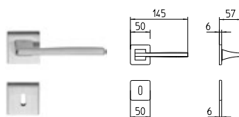
1031 MANIGLIA PER PORTA CON ROSETTA door-handle on rose
