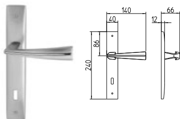
1140 MANIGLIA PER PORTA CON PIASTRA door-handle on back plate
