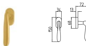
692/DK MARTELLINA DK drehkipp system
