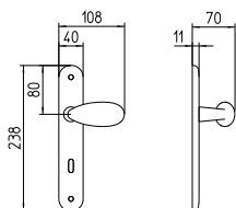
1090 MANIGLIA PER PORTA CON PIASTRA door-handle on back plate
