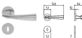
1141 MANIGLIA PER PORTA CON ROSETTA door-handle on rose
