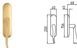
732/M CREMONESE IMPUGNATURA MANIGLIA window lever-handle
