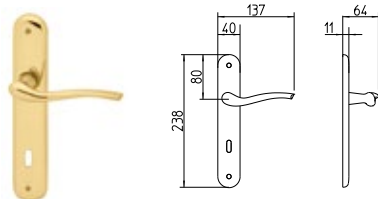
S70 MANIGLIA PER PORTA CON PIASTRA door-handle on back plate
