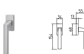
1292/DK MARTELLINA DK drehkipp system
