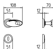
1111 MANIGLIA PER PORTA CON ROSETTA door-handle on rose
