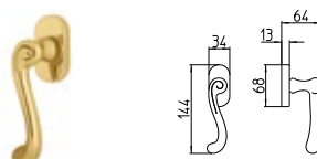
442/DK MARTELLINA DK drehkipp system
