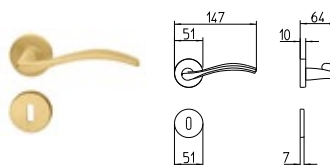
711 MANIGLIA PER PORTA CON ROSETTA door-handle on rose
