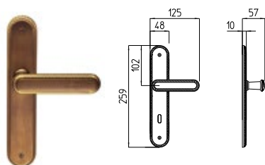
1640 MANIGLIA PER PORTA CON PIASTRA door-handle on back plate
