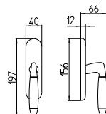
462/M CREMONESE IMPUGNATURA MANIGLIA window lever-handle
