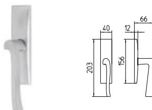
1072/M CREMONESE IMPUGNATURA MANIGLIA window lever-handle
