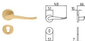
731 MANIGLIA PER PORTA CON ROSETTA door-handle on rose
