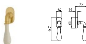
642/DK MARTELLINA DK drehkipp system
