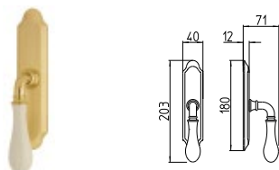
642/M CREMONESE IMPUGNATURA MANIGLIA window lever-handle
