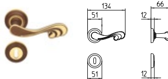
1121 MANIGLIA PER PORTA CON ROSETTA door-handle on rose
