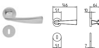
1131 MANIGLIA PER PORTA CON ROSETTA door-handle on rose
