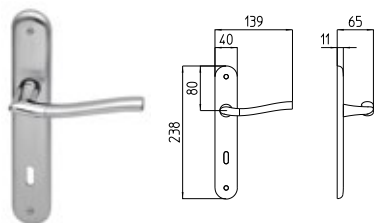
1180 MANIGLIA PER PORTA CON PIASTRA door-handle on back plate
