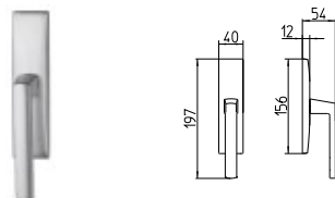
1292/M CREMONESE IMPUGNATURA MANIGLIA window lever-handle
