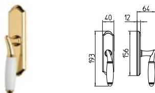
1202/M CREMONESE IMPUGNATURA MANIGLIA window lever-handle
