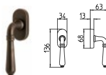
532/DK MARTELLINA DK drehkip system
