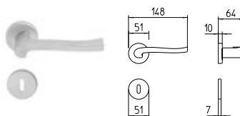
1071 MANIGLIA PER PORTA CON ROSETTA door-handle on rose
