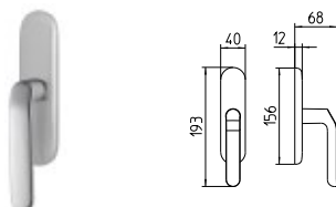
1612/M CREMONESE IMPUGNATURA MANIGLIA window lever-handle
