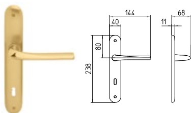
720 MANIGLIA PER PORTA CON PIASTRA door-handle on back plate
