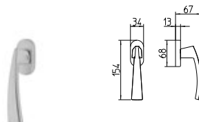
1132/DK MARTELLINA DK drehkipp system
