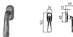
1442/DK MARTELLINA DK drehkipp system
