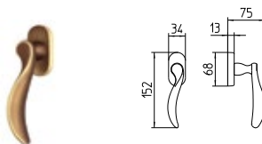
1212/DK MARTELLINA DK drehkipp system
