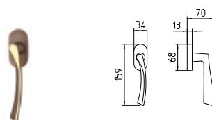
1472/DK MARTELLINA DK drehkipp system
