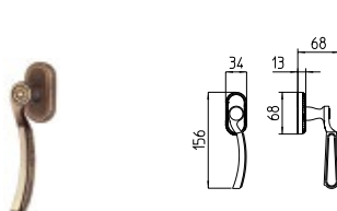
1412/DK MARTELLINA DK drehkipp system
