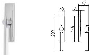
3182/M CREMONESE IMPUGNATURA MANIGLIA window lever-handle
