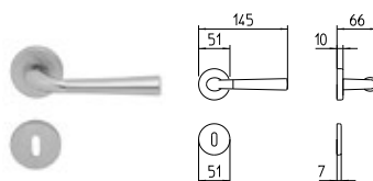
S101 MANIGLIA PER PORTA CON ROSETTA door-handle on rose
