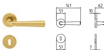
S91 MANIGLIA PER PORTA CON ROSETTA door-handle on rose
