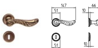
1661 MANIGLIA PER PORTA CON ROSETTA door-handle on rose
