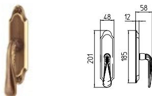
1432/M CREMONESE IMPUGNATURA MANIGLIA window lever-handle
