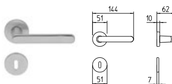
1301 MANIGLIA PER PORTA CON ROSETTA door-handle on rose
